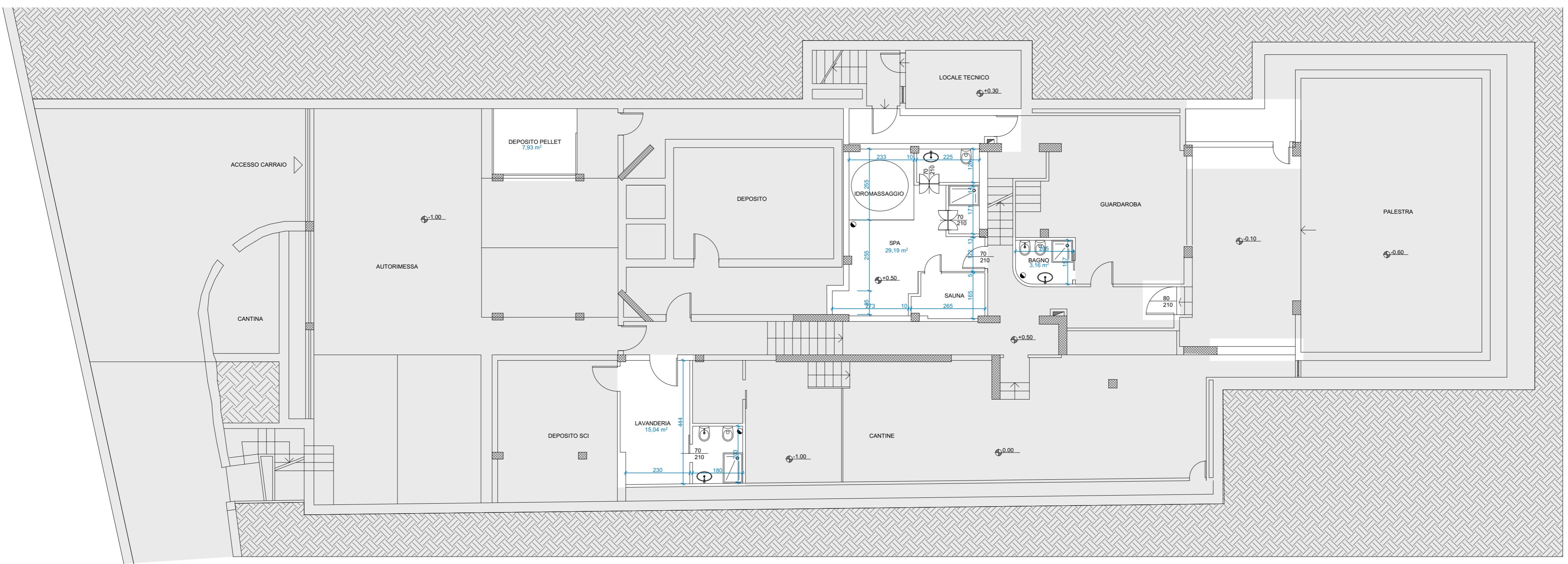
PIANO INTERRATO - STATO ATTUALE
