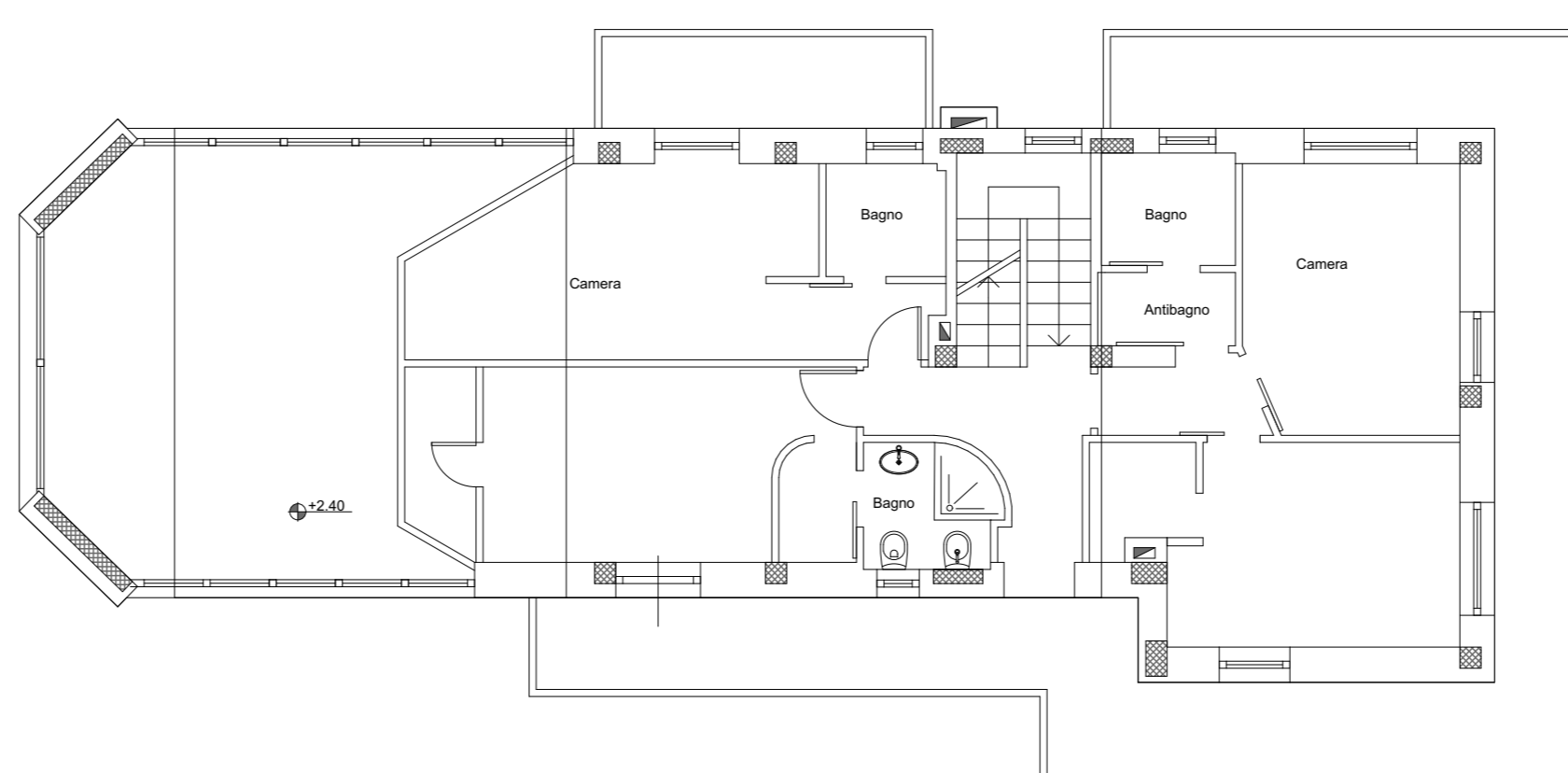
PIANO PRIMO - STATO ATTUALE
